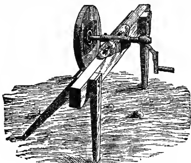
Fig. 71.—GRINDSTONE FRAME.
