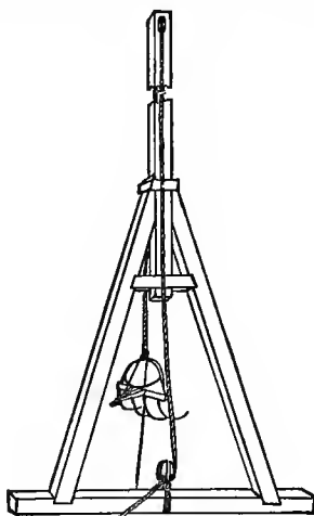
Fig. 153.—HAY DERRICK.
